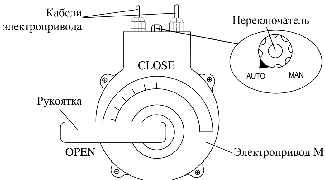
Рисунок 1.15 – Электропривод аварийного отсечного крана (вид сбоку)
