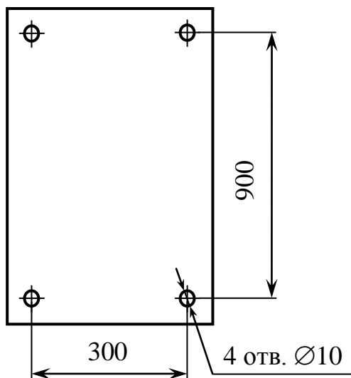
Рисунок 2.1 – Расположение отверстий для крепления панели всех исполнений УПП
