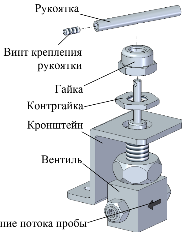
Рисунок 2.4 – Монтаж вентиля V1_{доп}
