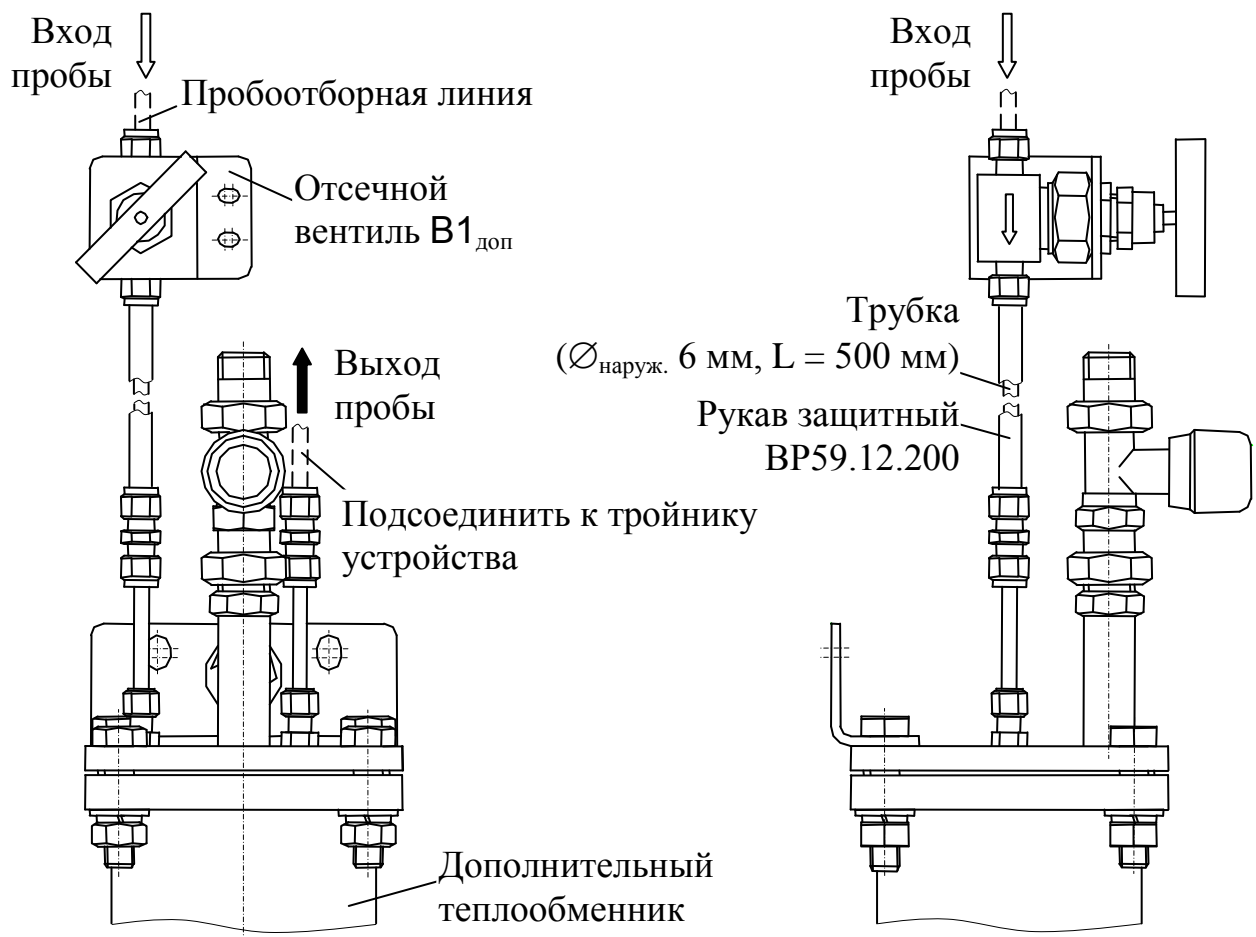
Рисунок 2.9 – Дополнительный теплообменник с входным вентилем
