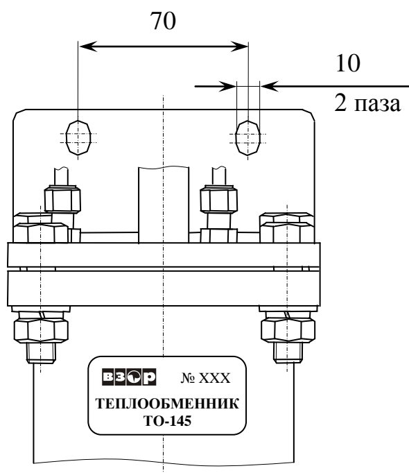
Рисунок 2.2 – Расположение отверстий на кронштейне крепления дополнительного теплообменника
