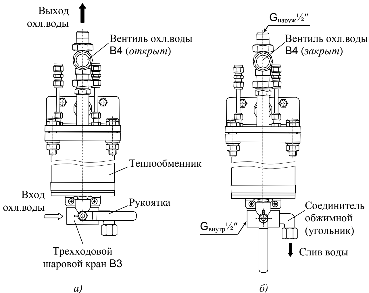
Рисунок 2.10 – Подача охлаждающей воды к теплообменникам (а), слив охлаждающей воды из теплообменников (б)
