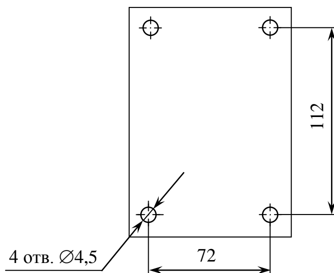
Рисунок 2.5 – Расположение отверстий для крепления источника питания ИП-01мк
