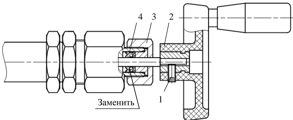
Рисунок 3.3 – Регулирующий вентиль (замена манжеты)
