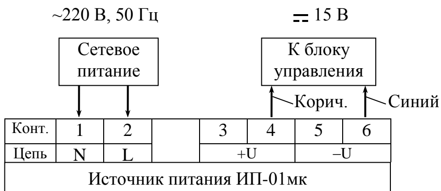
Рисунок 2.14 – Схема подсоединения кабелей к источнику питания ИП-01мк
