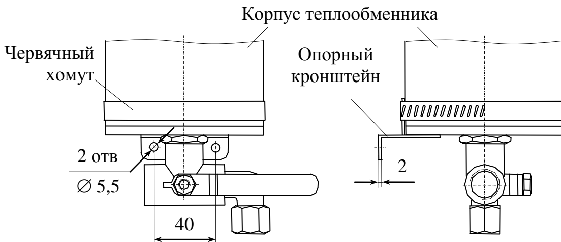
Рисунок 2.3 – Крепление дополнительного теплообменника
