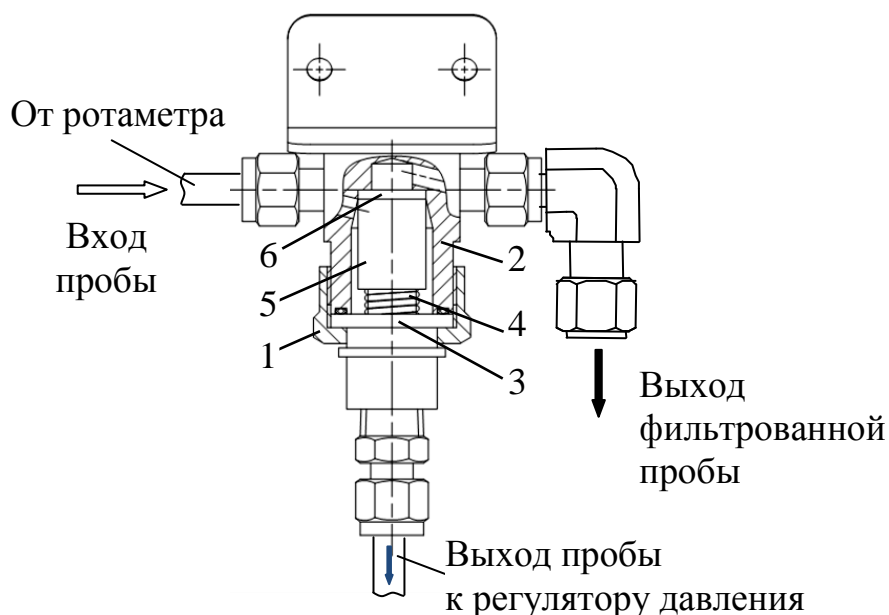
Рисунок 3.2 – Фильтр механической очистки
