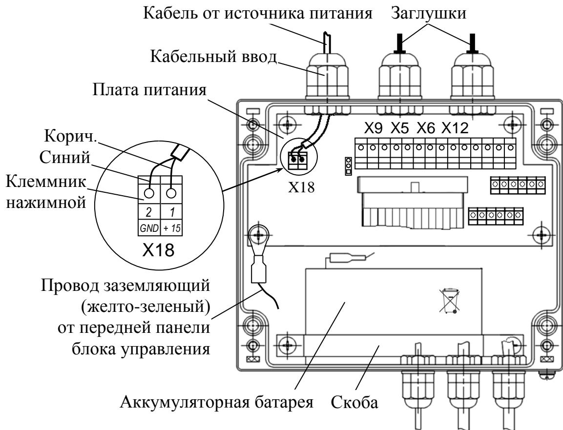
Рисунок 2.12 – Расположения контактных устройств для внешних подключений блока управления (вид без передней панели)
